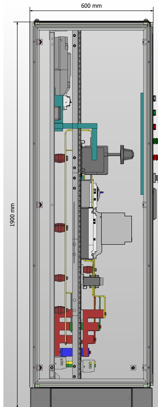
Вид слева
